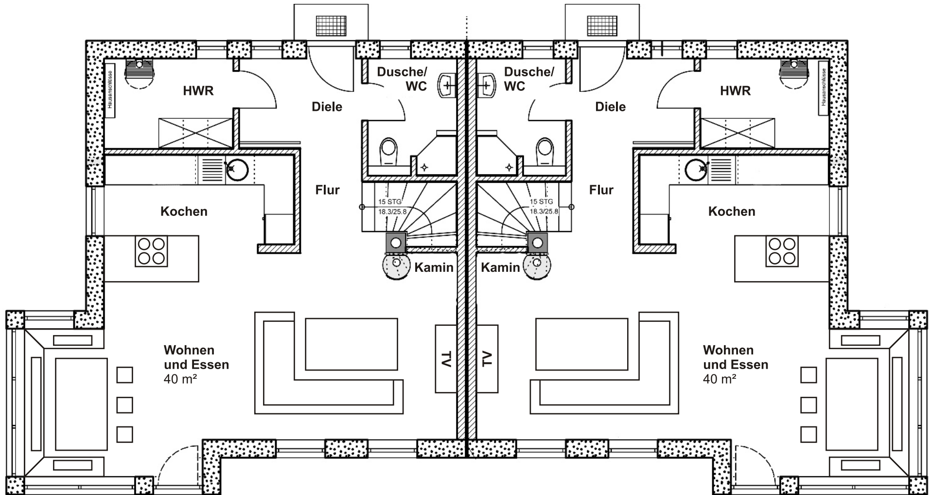
Erdgeschoss
