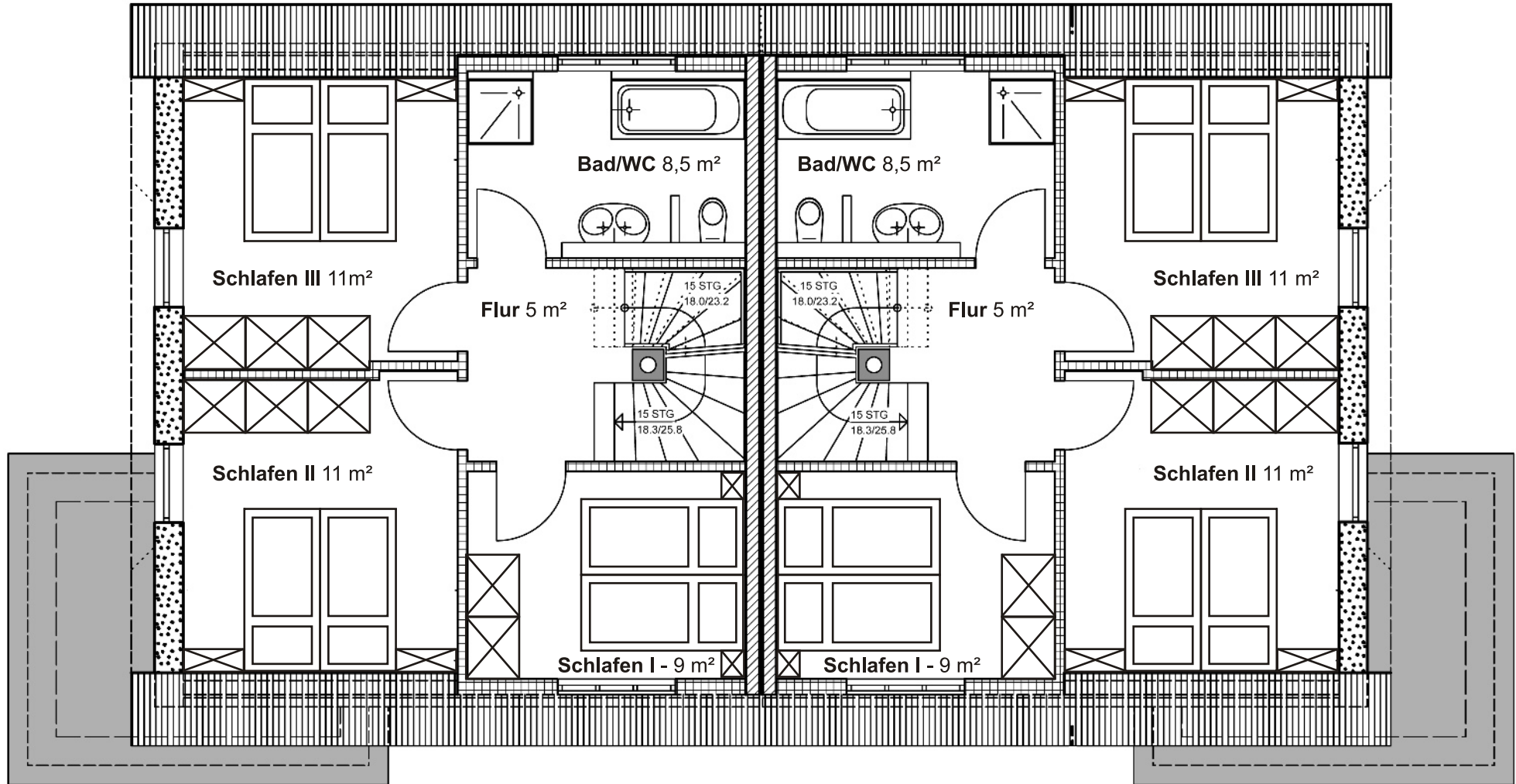
Dachgeschoss
